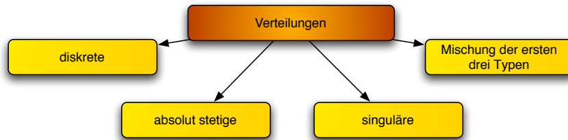
Abbildung 3.7: Verteilungstypen
