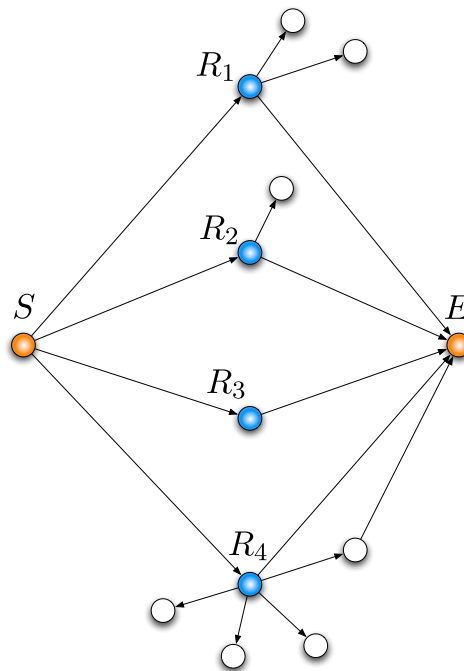
Abbildung 2.17: Routing-Problem: Computernetzwerk
