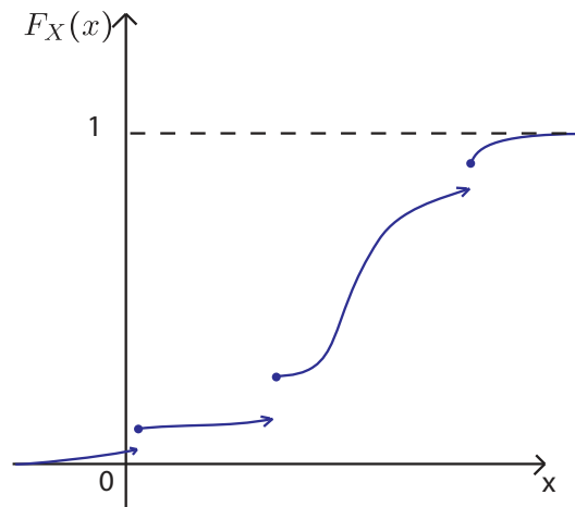
Abbildung 3.6: Typische Verteilungsfunktion
