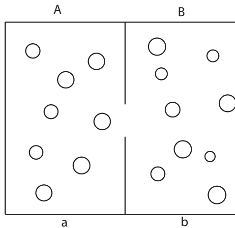
Abbildung 2.14: Diffusionsproblem
