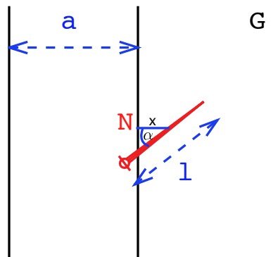
Abbildung 2.7: Buffonsches Nadelproblem
