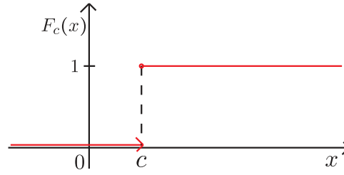
Abbildung 6.1: Verteilungsfunktion F_c
