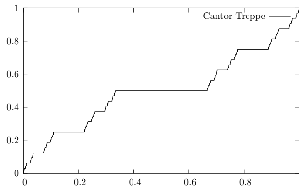
Abbildung 3.15: Cantor-Treppe
