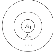
Abbildung 2.3: Mengenschachtelung
